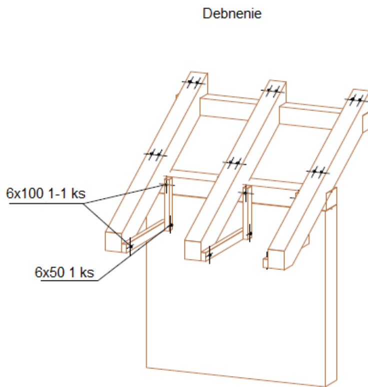
12. obrázok: Debnenie náčrt
