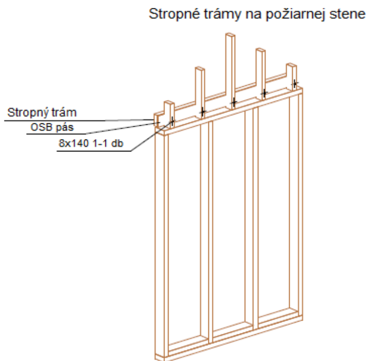
24. obrázok: Stropné trámy na požiarnej stene náčrt
