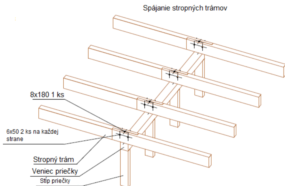
22. obrázok: Spájanie stropných trávov náčrt
