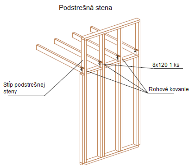
38. obrázok: Podstrešná stena náčrt
