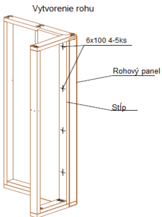
28. obrázok: Vytvorenie rohu náčrt
