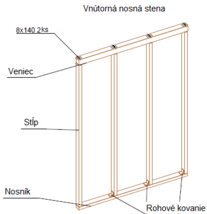
6. obrázok: Vnútorá nosná stena náčrt
