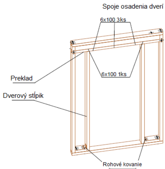
4. obrázok: Osadenie dverí náčrt
