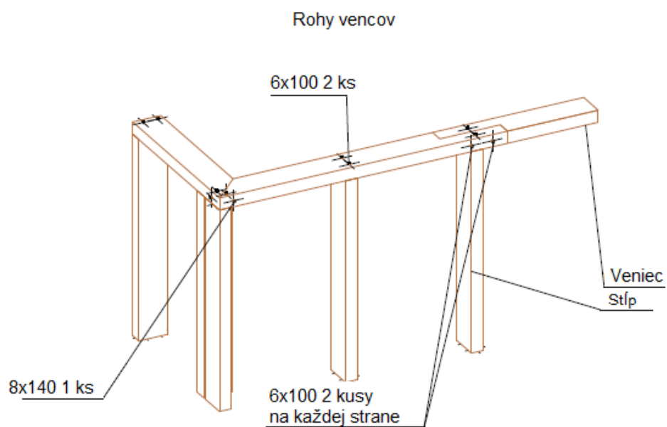
26. obrázok: Rohy venca + spoje náčrt
