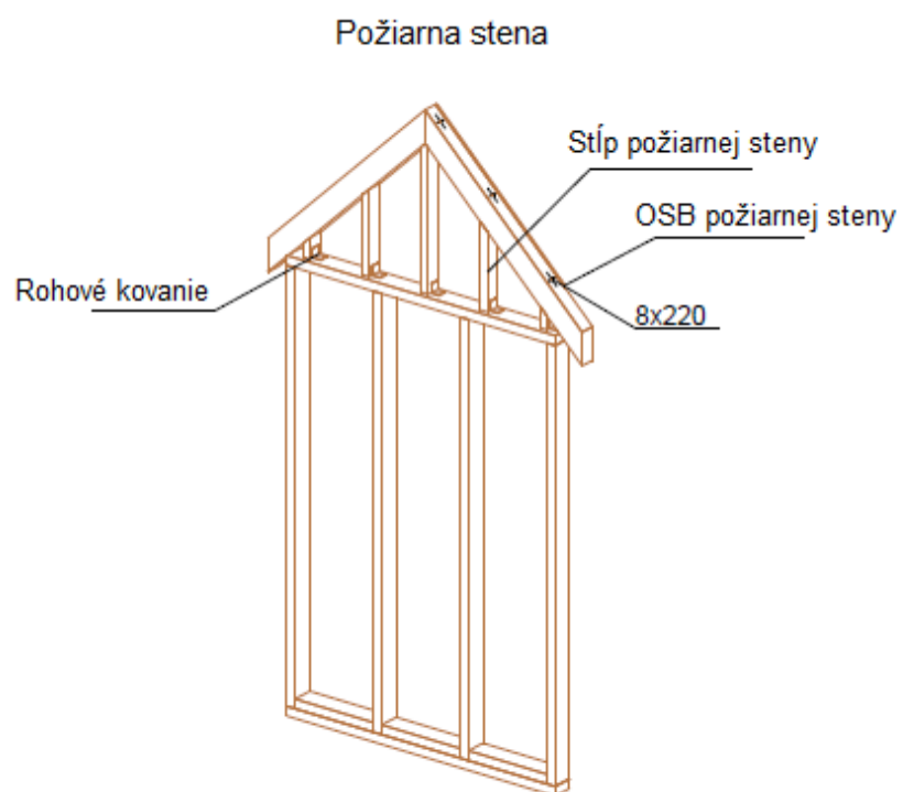
40. obrázok: Požiarna stena náčrt
